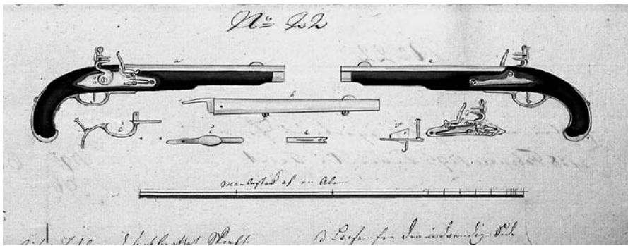
Husarpistol M1795. Den nye pistol, der godkendes i 1795, havde ikke ladestokken monteret i træet under løbet. Derudover var kolbekappen gjort længere for at forstærke kolben. Som på husarernes øvrige skydevåben var træet bejdsset sort. von Bergens våbenbog. Tøjhusmuseet.
