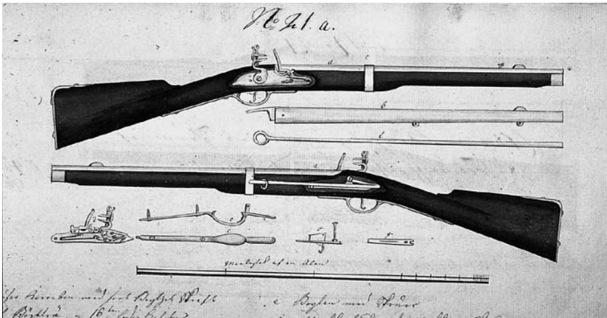
Husarkarabin M/1795. I forhold til den tidligere model var den mest synlige forskel, at ladestokken ikke længere skulle være monteret under løbet, men skulle bæres i en separat rem. von Bergens våbenbog. Tøjhusmuseet.
