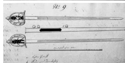
Rytterpallask M/1773 og den ganske let forandrede M/1778 havde begge skeder af træ med jernbeslag og tre bæringene. von Bergens våbenbog. Tøjhusmuseet.
